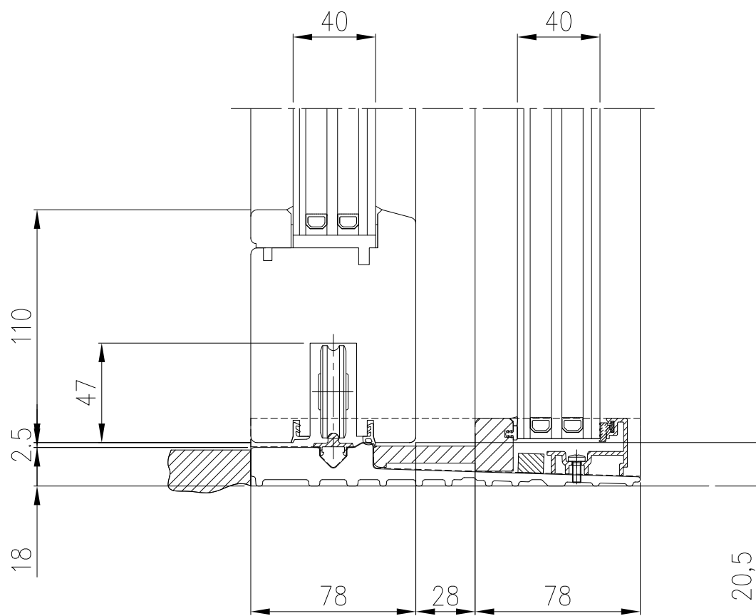
SEZIONE VERTICALE
