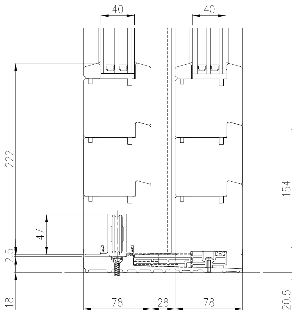
SEZIONE VERTICALE
