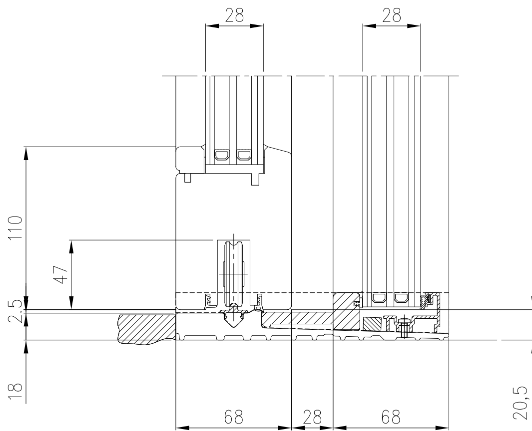
SEZIONE VERTICALE
