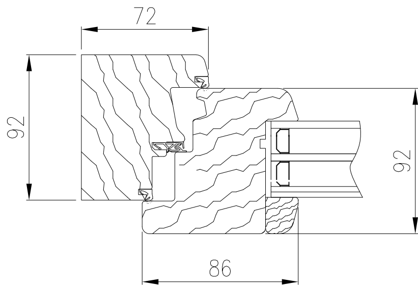
A Sez. nodo laterale / superiore
